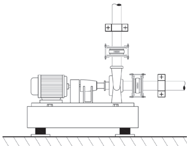
Instalación de Manguitos con tirantes
