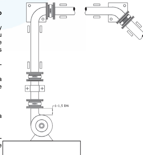
Instalación de Manguitos sin tirantes
