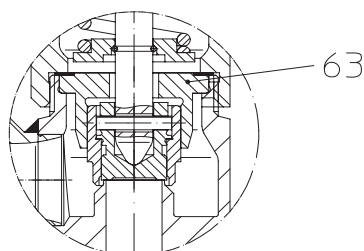
Cono BR950
