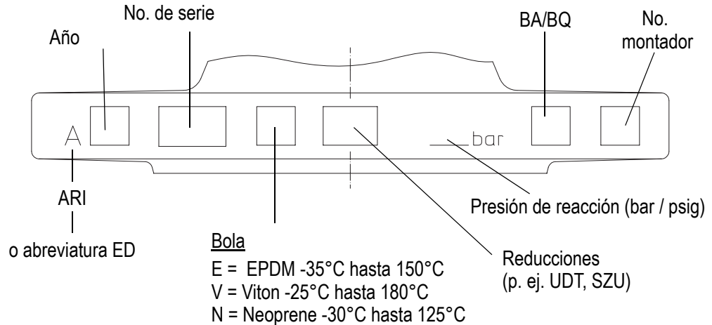
Fig. 4: Caja (brida de salida)
